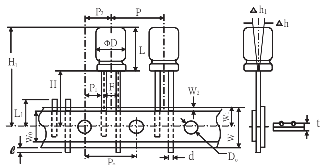
Fig.5(φ 12~φ 13)
