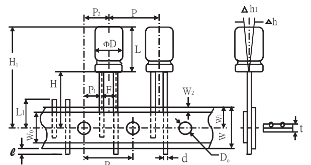
Fig.6(φ 16)
